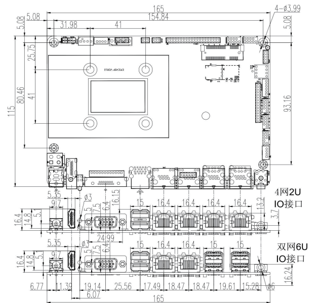
双网IO图
